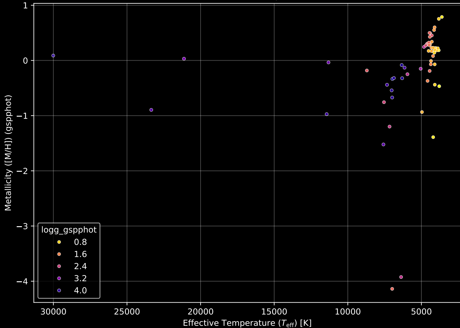
APOGEE DR17 Field: [279-35-O] Stellar Population Parameters (n= 59)
